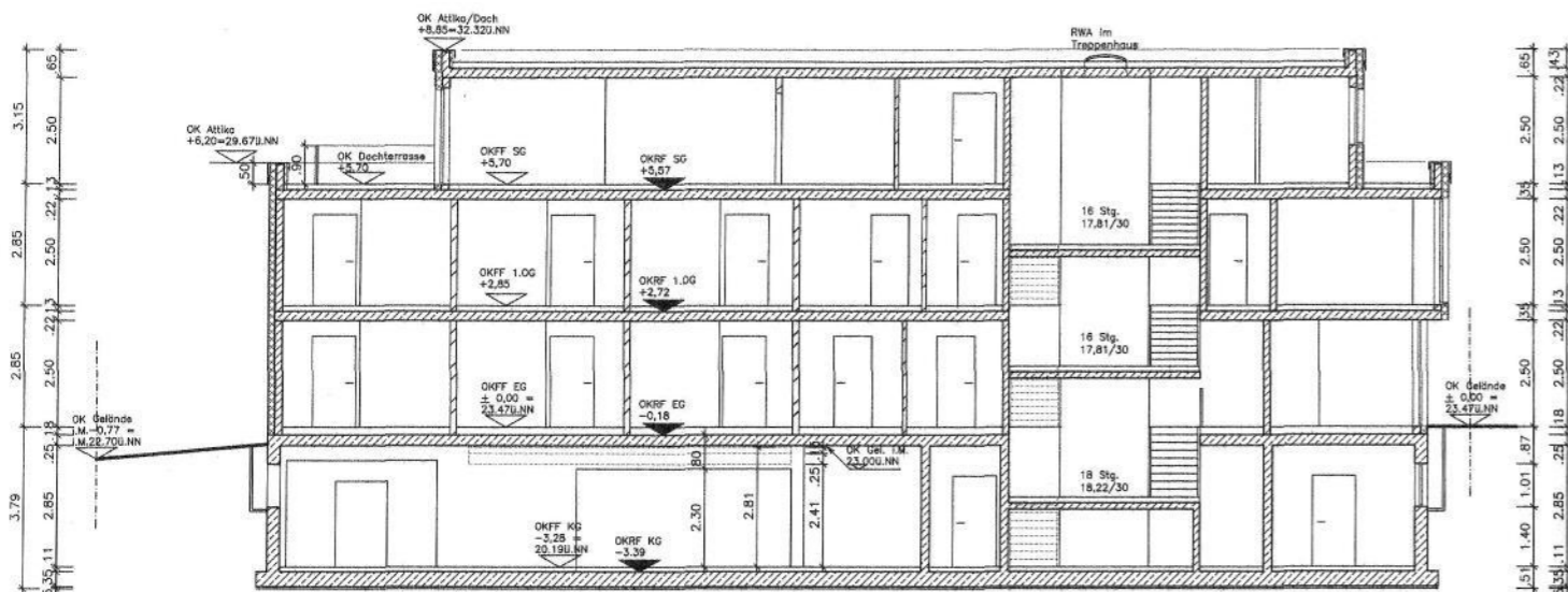
Schnitt A-A
