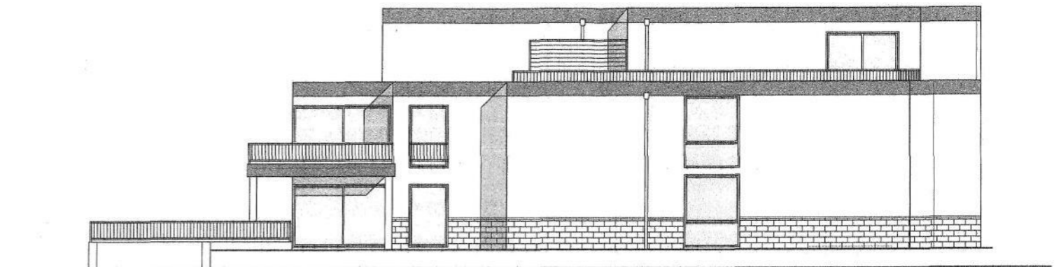
Ansicht Süd-Ost
